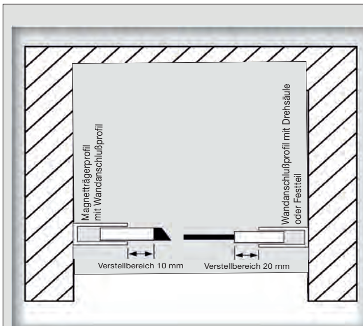
Anschlag rechts
